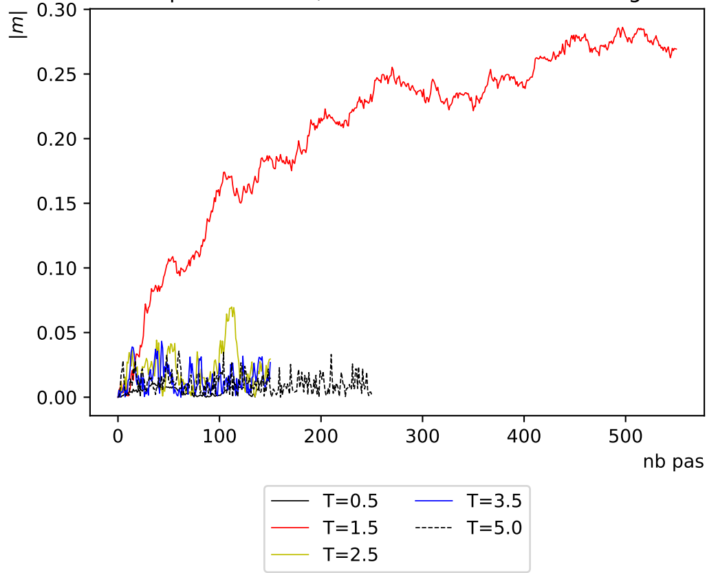
Evolution selon critère Estimation par intervalle,Condition Initiale alterné 4lignes-4lignes, Réseau taille L=128
